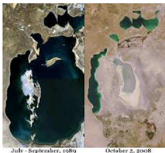
Рисунок 2 – Контуры Арала – методом космического зондирования (1989 г., 2008 г.)
