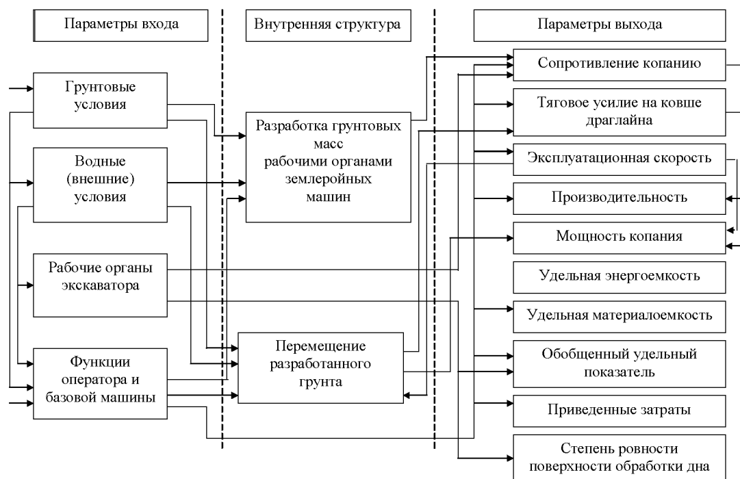
Структурная схема процесса копания грунта ковшем драглайна в подводных условиях
