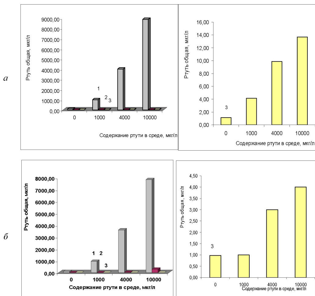
Рис. 2. Эффективность фильтрации на среде лактатом (а) и с ацетатом (б). 1 – фильтр «синяя лента»; 2 – мембранный фильтр; 3 – фильтр
