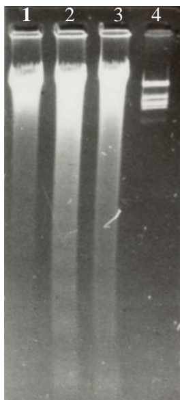
Рис. 4. Электрофореграмма ДНК клеток ХАО КЭ, зараженных различными вирусами в разведении 10^{-5} , 12 ч.
