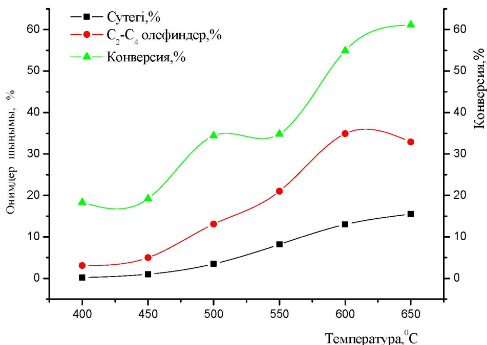
2-сурет. Mn-Cr(1/1)/SiO 2 -катализаторында пропан конверсиясына, олефиндер мен суреті шыңымына температураның әсері ( t_{\text{актив}} = 550^{\circ}\text{C} , V_{\text{кол}} = 600 \text{ саң}^1 , P_{\text{H}_2\text{O}} = 0,19 \text{ атм} )
