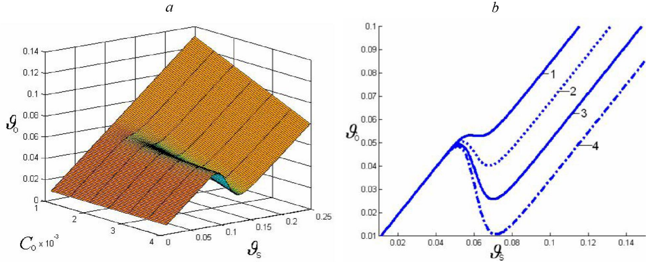
Fig. 1. Bifurcation set (a) and bifurcation diagram (b): a - G_0 = 0,025; Pe = 130; Pe_c = 130; Da = 1,7 \cdot 10^9; Bi_T = 2; Bi_{T_c} = 2; q = 16,7; b - C_0 = 0,001 (1); 0,002 (2); 0,003 (3); 0,004 (4)
