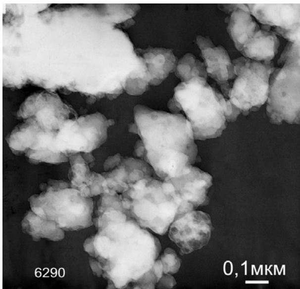
Рис.3. Электронно-микроскопический снимок. Морфология рыхлых комковатых и округлых «пузырчатых» частиц криптокристаллического образования каратауитового состава (обр. М-13). Месторождение Баласаускандык. Электронный микроскоп JEM-100CX, ускоряющее напряжение 100 кВ). Аналитик Т. А. Шабанова
