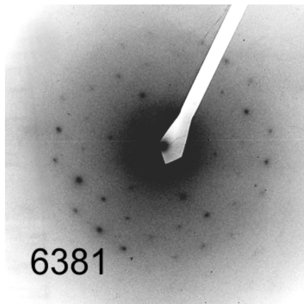
Рис. 4. Точечная электронограмма от слоистой частицы криптокристаллического образования каратауитового состава (обр. М-13). Месторождение Баласаускандык. Электронный микроскоп JEM-100CX, ускоряющее напряжение 100 кВ. Аналитик Т.А.Шабанова
