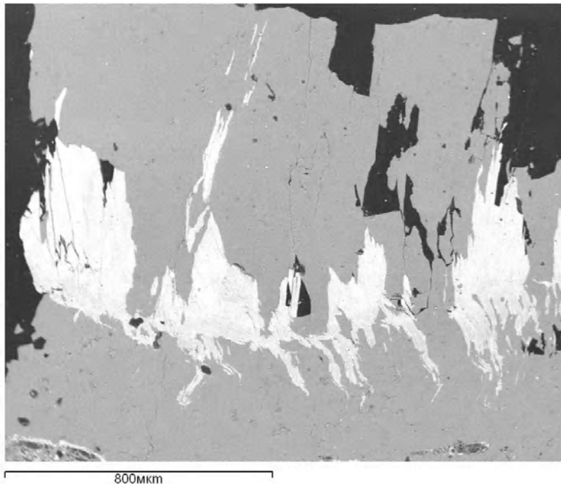
Рис. 2. Кварц-роскоэлитовый прожилок. Бариевый роскоэлит (белое) прорастает шестоватый кварц (серое), залечивая срединный шов прожилка. Месторождение Баласаускандык. Изображение полированной поверхности в обратнорассеянных электронах (состав). Аналитик П. Е. Котельников
