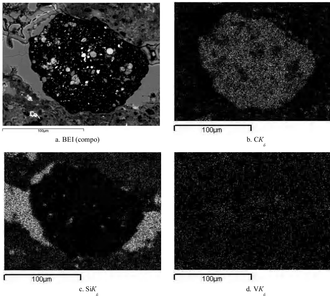
Рис. 1 а. Округлое образование ОБ (черное) в кремнистом (серое) материале пород пачки. Месторождение Курумсак. Изображение полированной поверхности в обратнорассеянных электронах (состав): b–d. То же в рентгеновском характеристическом излучении элементов. Аналитик П. Е. Котельников
